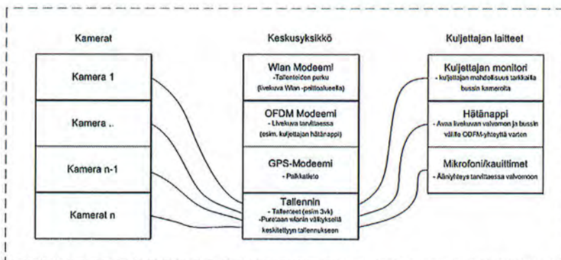
Kuva 6 Turvakamerajärjestelmän lohkokkaavio (yleinen esitys).
